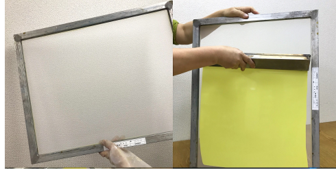
型枠 乳剤を流し塗布する
